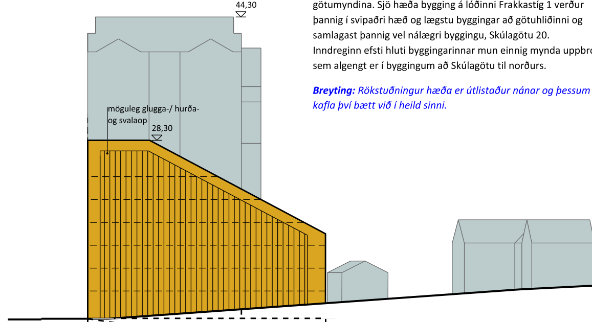
SNEIÐING A-A, TILLAGA AÐ DEILISKIPULAGSBREYTINGU, 25.5.2018, SEM VAR SÍÐAR FELD ÚR GILDI, mkv. 1:500
