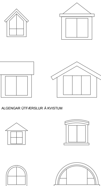
MYND 7 Mismunandi gerðir kvista.
